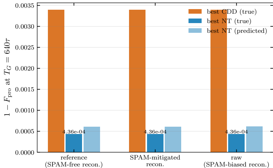
(d) idle: SPAM-arm designs ( T_G = 640\tau )
