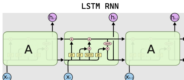
Figura 5.1: Ejemplo de una arquitectura RNN-LSTM [5]
