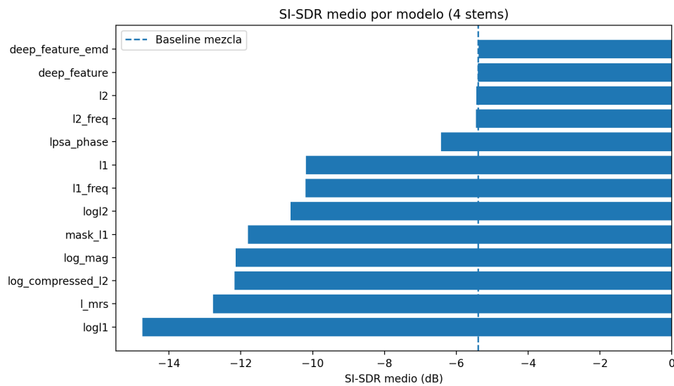
Figura 8.2: Gráfico de barras de los valores SI-SDR de cada función de pérdida en la separación de cuatro fuentes
