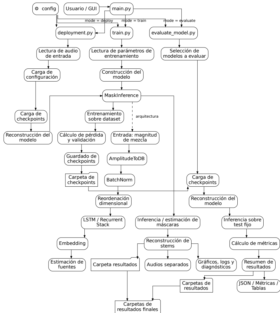
Figura 7.1: Diagrama de flujo para el backend
