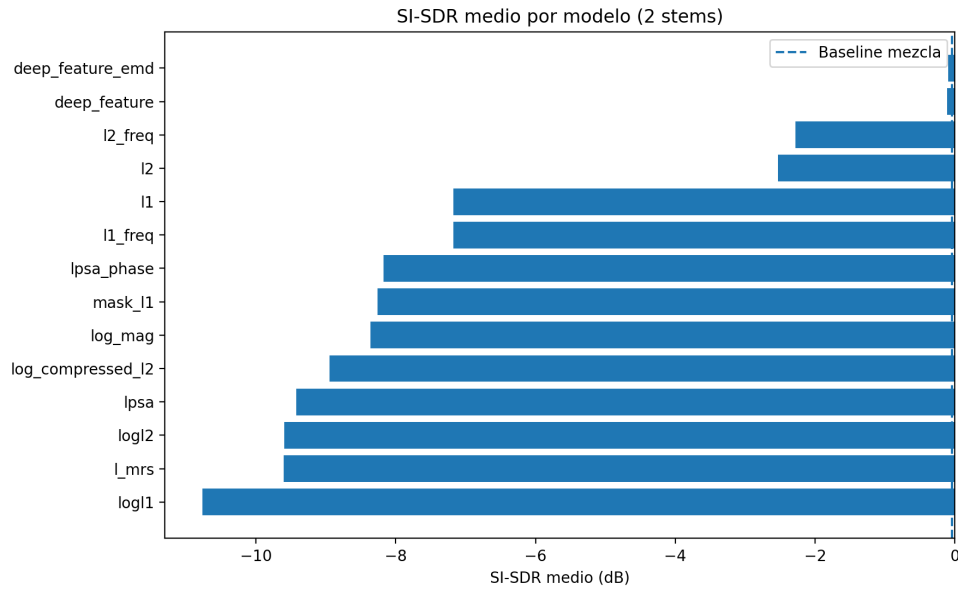
Figura 8.1: Gráfico de barras de los valores SI-SDR de cada función de pérdida en la separación de dos fuentes
