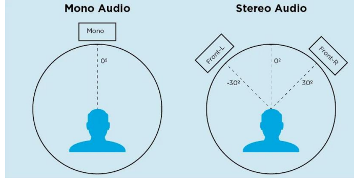
Figura 4.5: Representación gráfica de las diferencias entre sonido mono y sonido estéreo.
