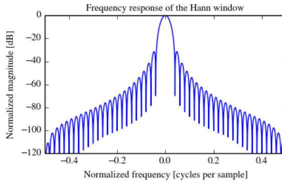
Figura 4.7: Respuesta frecuencial de una ventana Hann.
