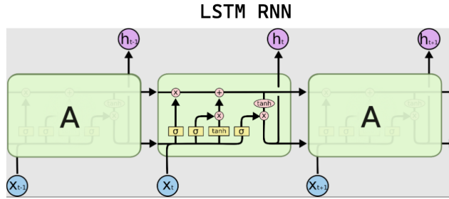
Figura 6.1: Ejemplo de una arquitectura RNN-LSTM [6]
