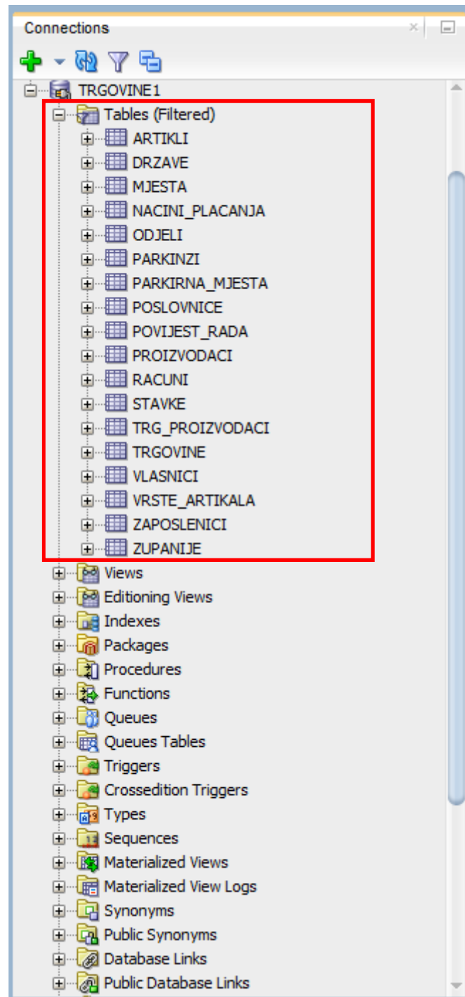
Slika 8. Tablice baze podataka
