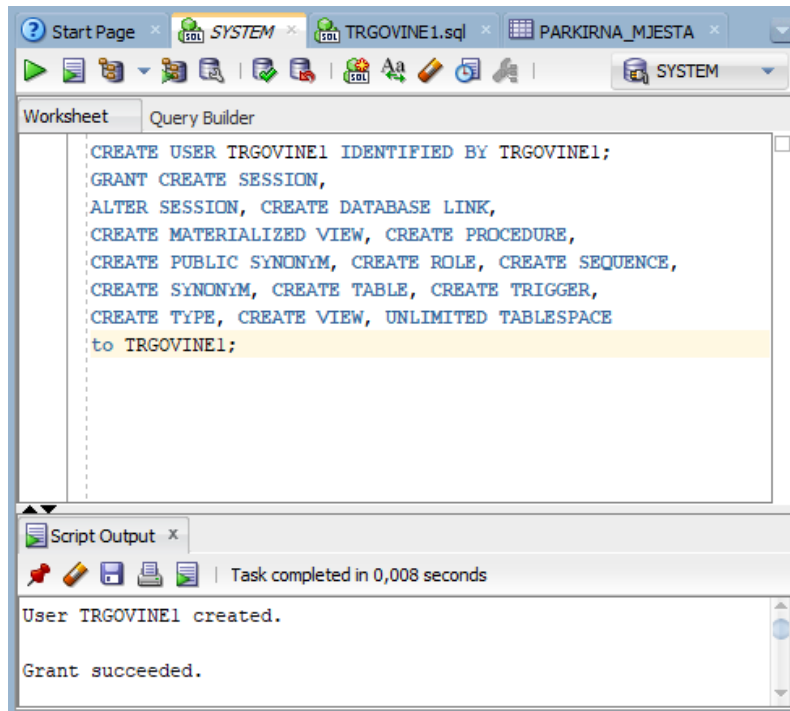
Slika 6. Kreiranje korisnika te dodjeljivanje ovlasti
