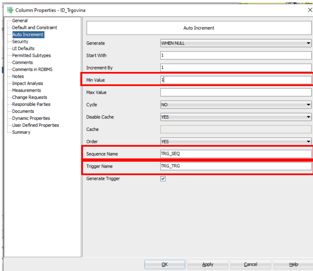
Slika 4. Sekvenca i trigger
