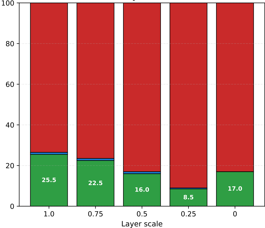
CodeGen-NL Layer 11
