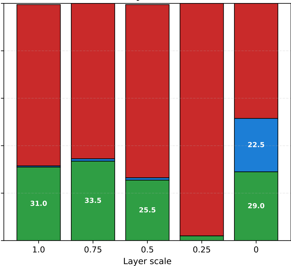
CodeGen-Mono Layer 13
