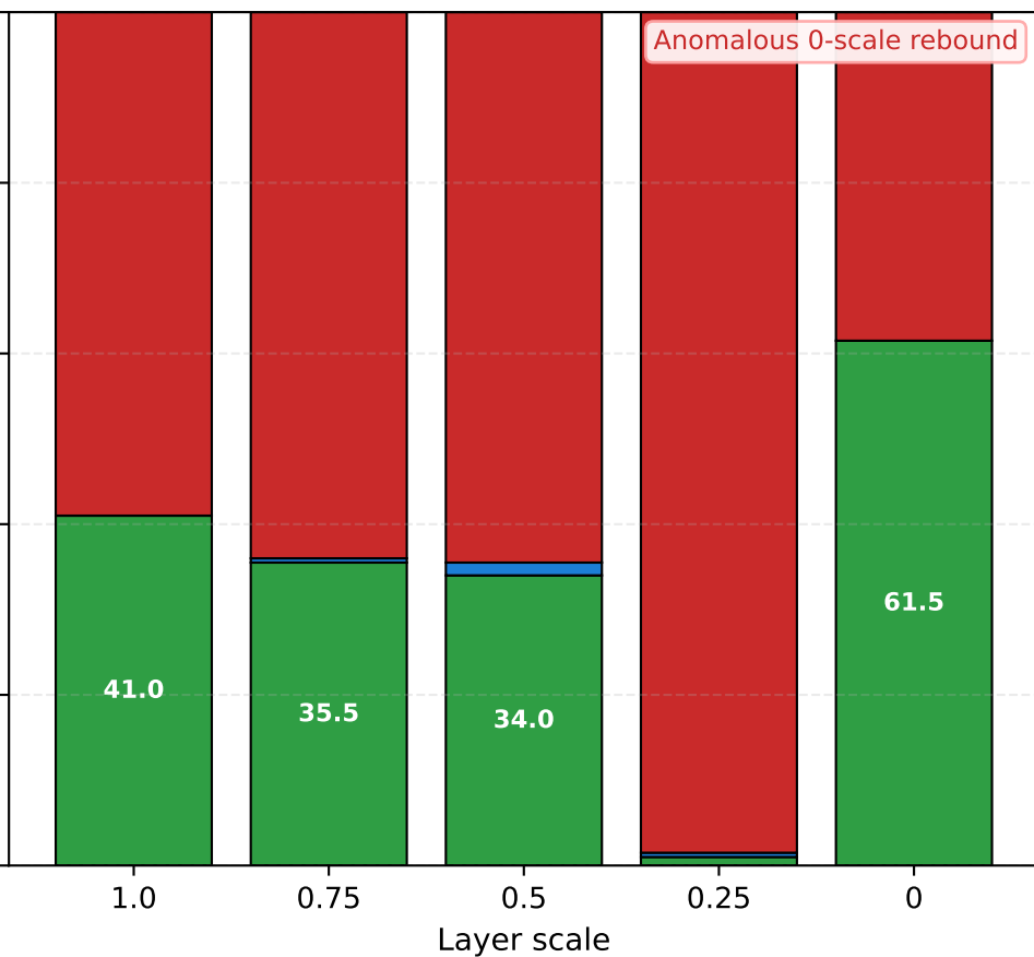
CodeGen-Multi Layer 7 Anomalous 0-scale rebound
