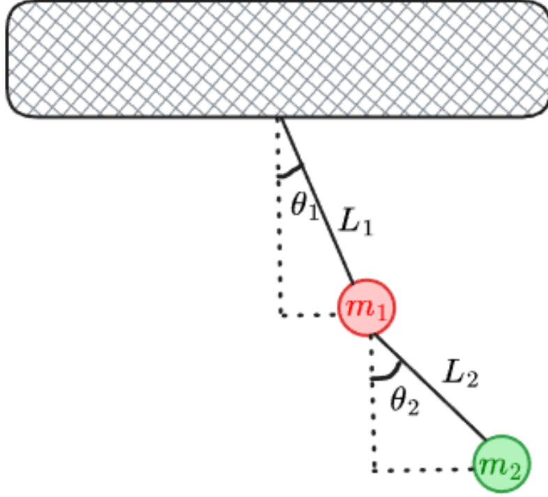
Figure 2: Schéma d'un double pendule. Le support en gris hachuré est fixe. La masse m_1 est relié au support par une corde de taille fixe L_1 . La masse m_2 est reliée à la masse m_1 par une corde de taille fixe L_2 .
