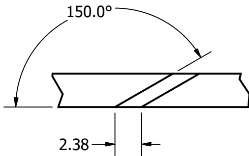
DETALLE A ESCALA 3 : 1
