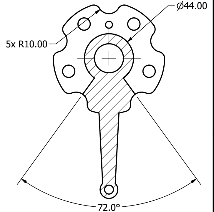
SECCIÓN B-B
