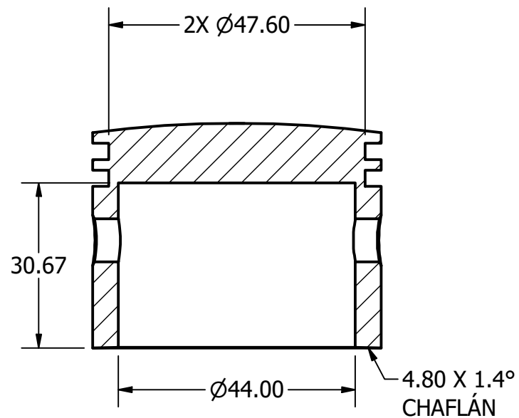
SECCIÓN A-A ESCALA 1 : 1
