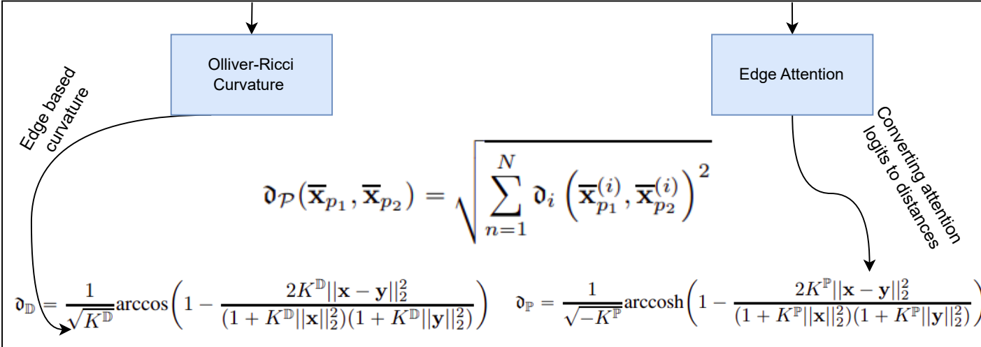
Edge Attention Module
