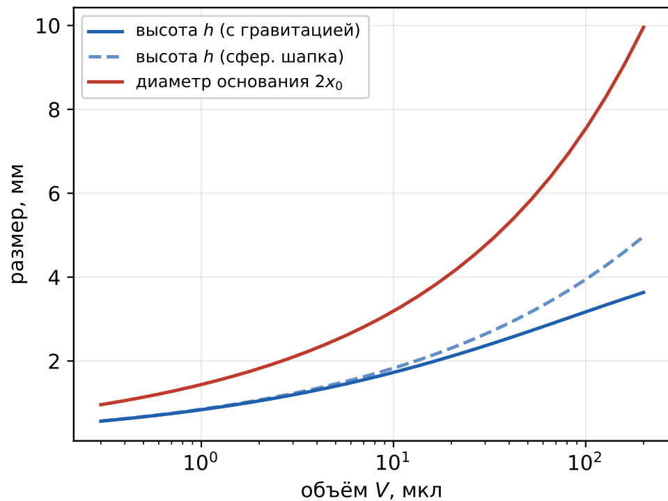
Отклонение от сферической шапки с ростом V
