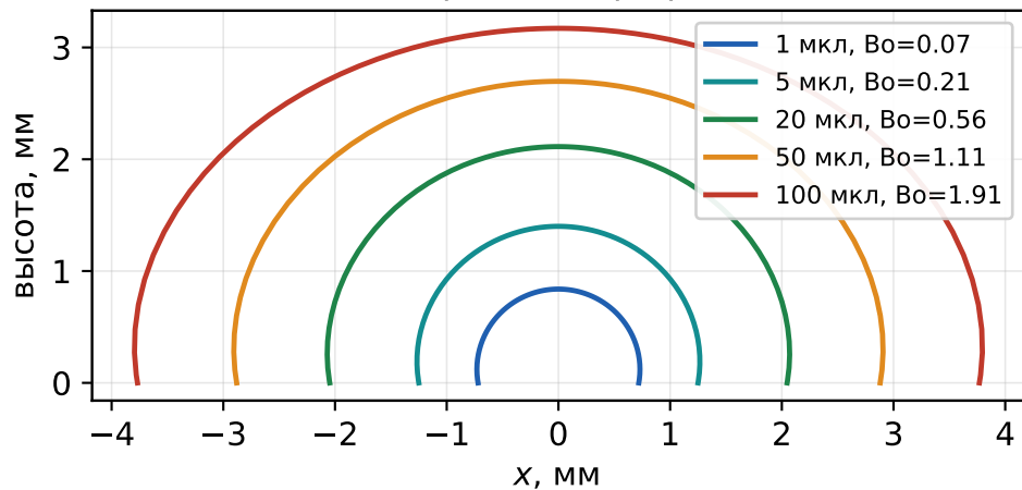
Осесимметричные профили (вода)
