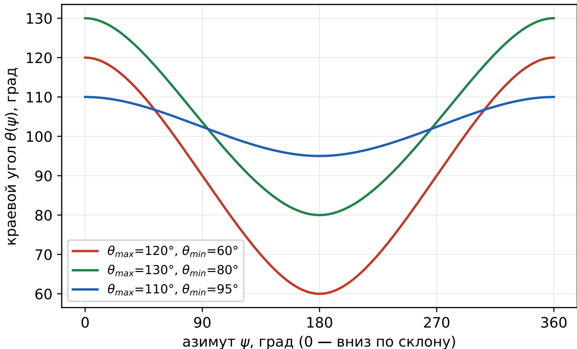
Распределение краевого угла по периметру (кубика, ElSherbini)
