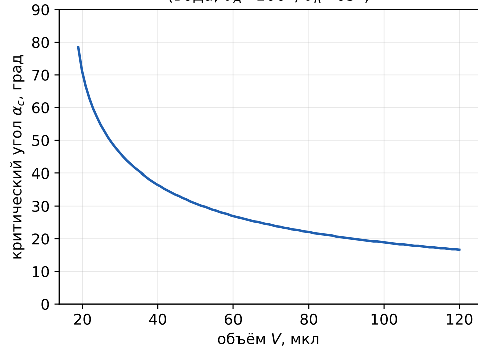
Угол начала соскальзывания (вода, \theta_A=100^\circ , \theta_R=65^\circ )
