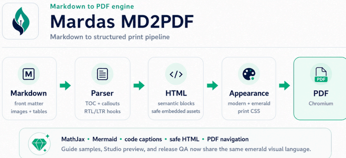
شکل ۱. نمای کلی معماری.
