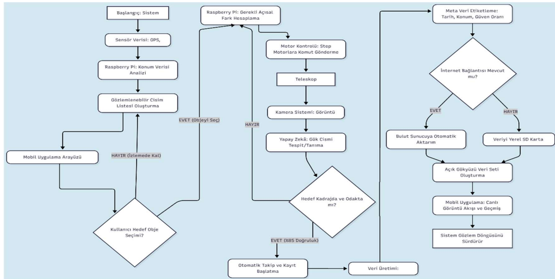
Şekil 5. Otonom Teleskop Sisteminin Genel Akış Diyagramı
