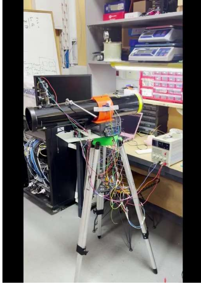
Şekil 6. Bütçe dostu prototipin sahaya kurulmuş hâli
