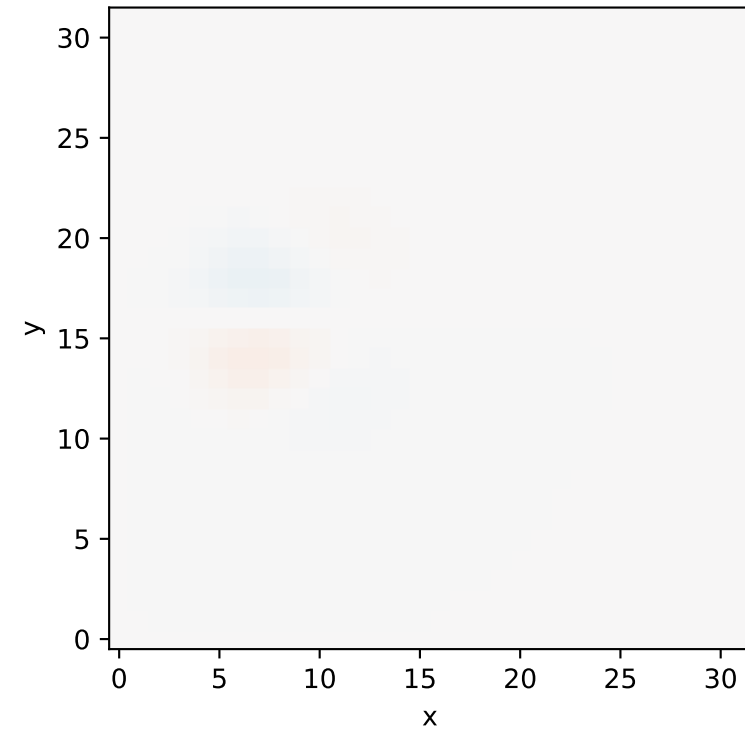
RK4 (dt=0.01)
