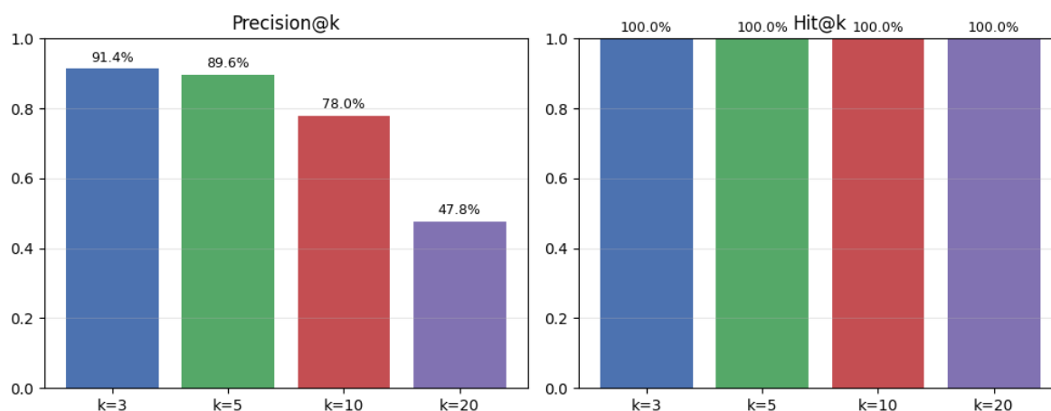
Рисунок 2.5 – Метрики итоговой конфигурации #5: precision@ k и hit@ k для k \in \{3, 5, 10, 20\}
