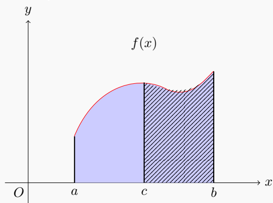
Рис. 3.1. Интегралы с переменными верхними пределами
