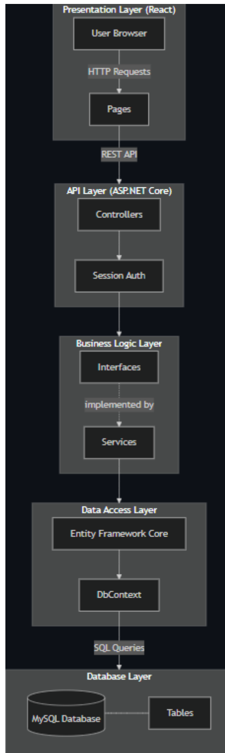
15. ábra: Alkalmazás architektúra
