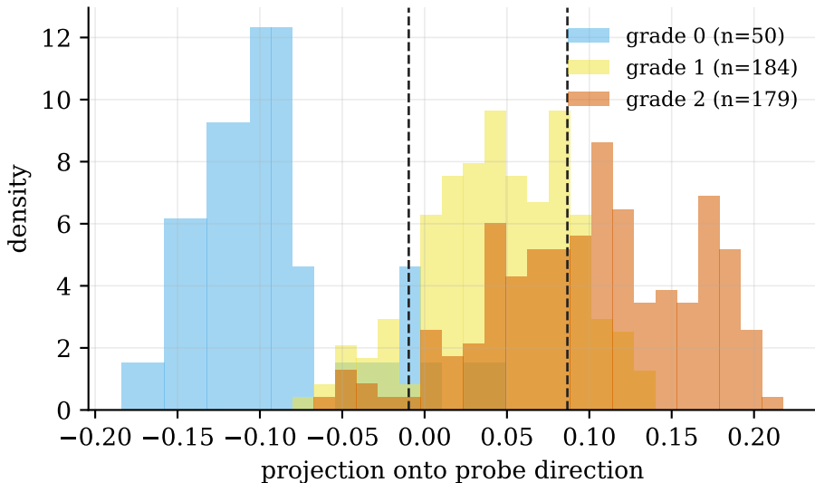
ET — gemini/generic (TEST macro-F1=0.70)
