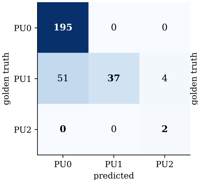
gpt-oss-safeguard-20b
