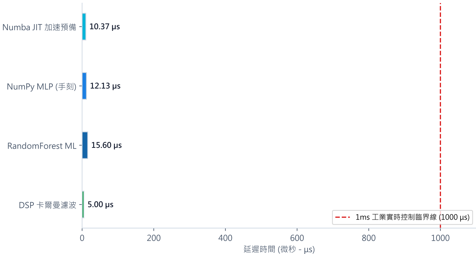
邊緣端演算法單次推理延遲對比 (μs)
