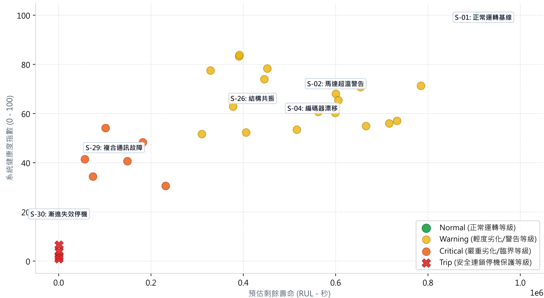
30 個伺服故障情境之「健康度 - 剩餘壽命 (RUL)」分佈軌跡圖
