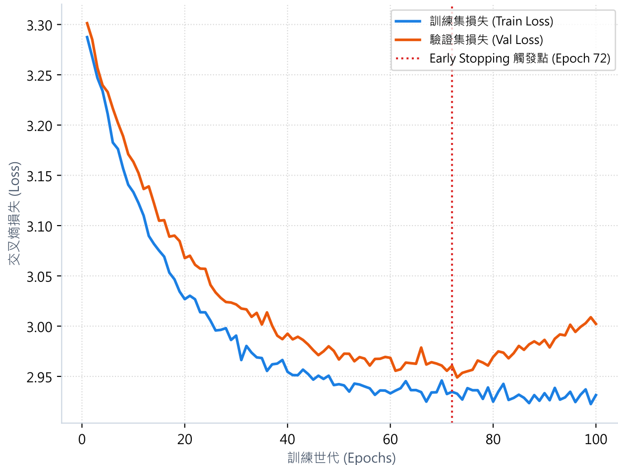
手刻 AutogradMLP 訓練收斂與早停監控
