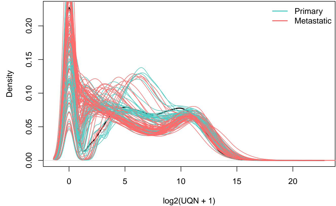
Densidad de expresión
