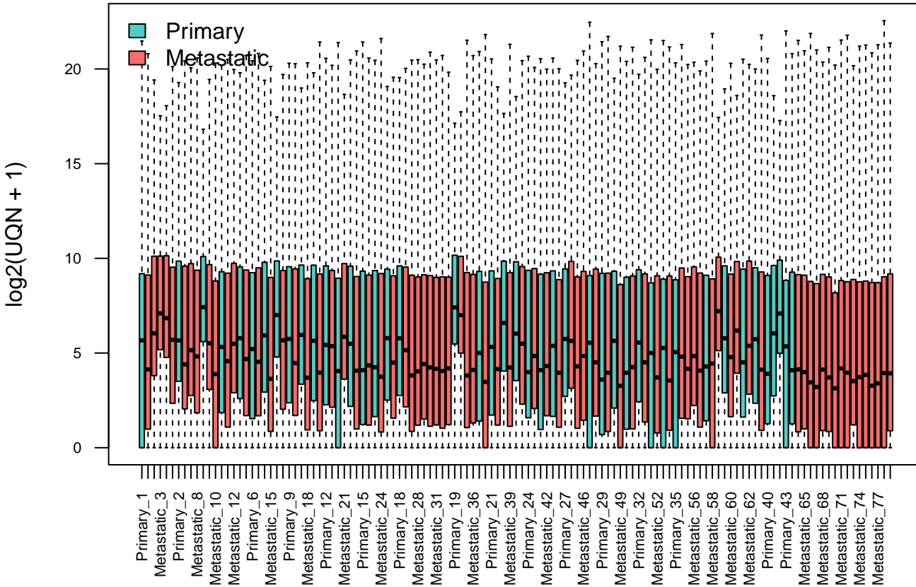
Distribución \log_2(\text{UQN}+1) por muestra
