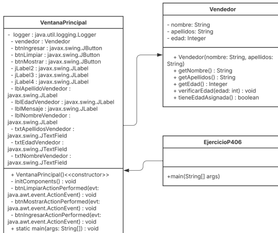
Figura 4: Diagrama de clases (UML) ejercicio P406
