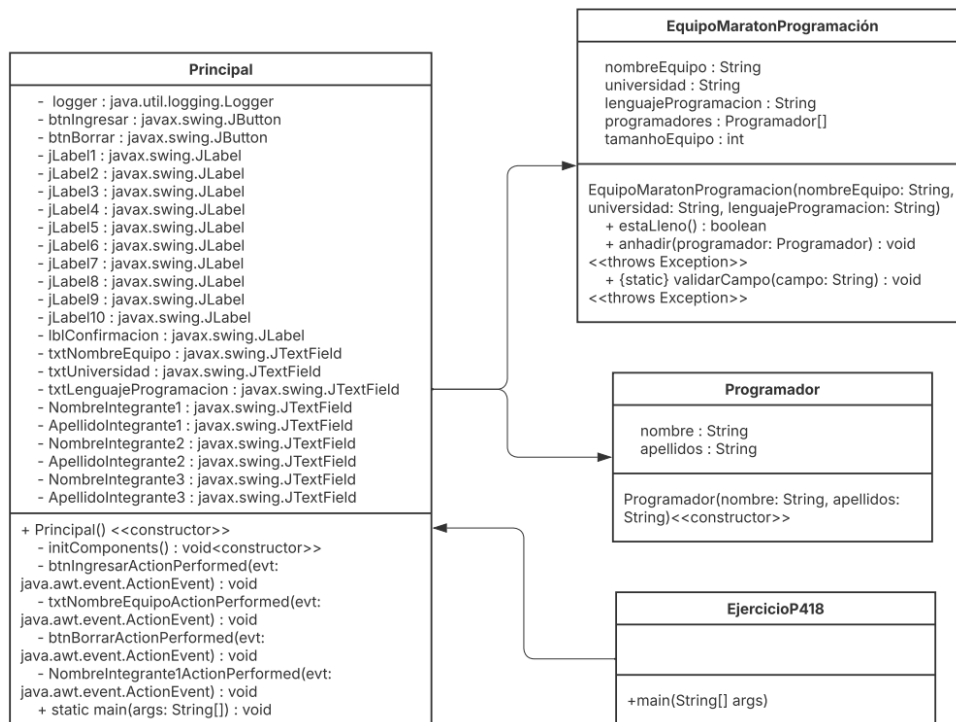
Figura 10: Diagrama de clases (UML) ejercicio P418
