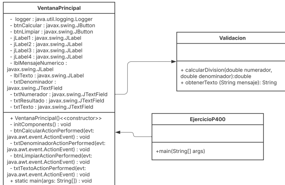
Figura 1: Diagrama de clases (UML) ejercicio P400
