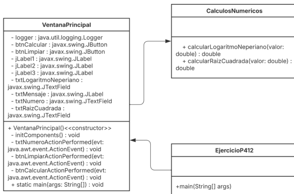
Figura 7: Diagrama de clases (UML) ejercicio P412
