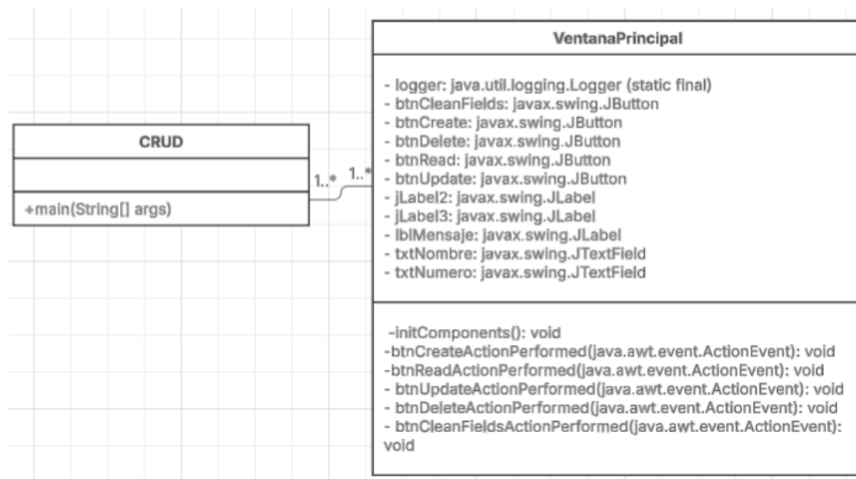
Figura 2: Diagrama de clases (UML) - Sistema CRUD
