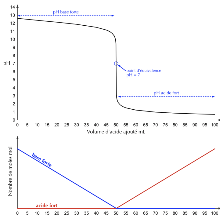
FIGURE 18.6 – Neutralisation d'une base forte par un acide fort
