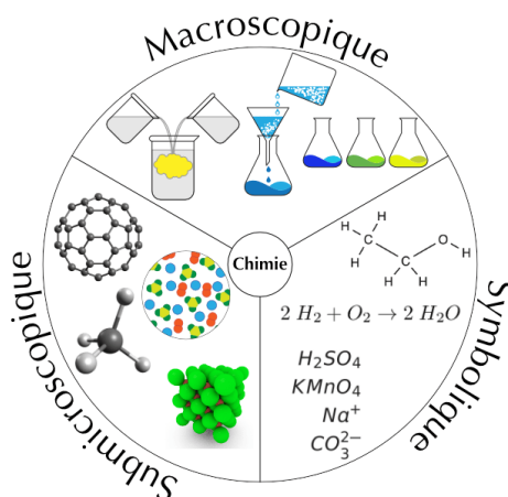
FIGURE 2.1 – Les trois niveaux de représentation de la chimie
