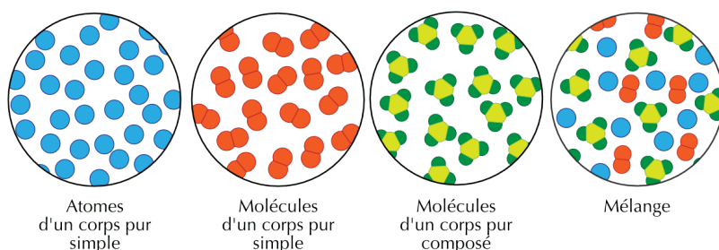
FIGURE 3.1 – Corps purs et corps composés
