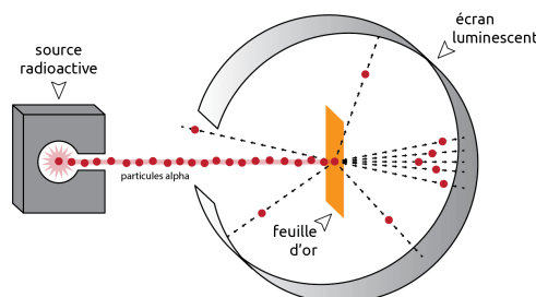
FIGURE 4.3 – Bombardement de la feuille d'or
