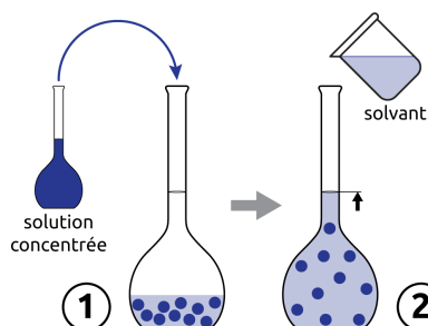
FIGURE 10.9 – Préparation d'une solution par dilution
