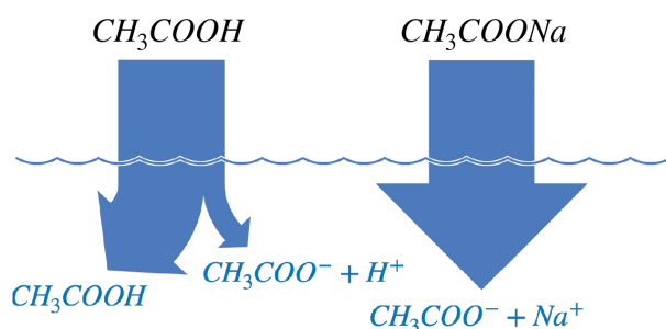
FIGURE 18.2 – Solution tampon acide acétique / acétate de sodium
