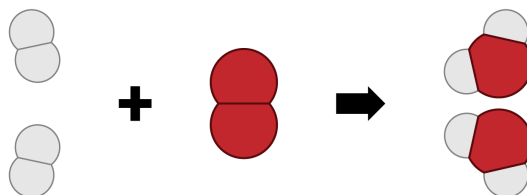
FIGURE 11.1 – Exemple de réaction
