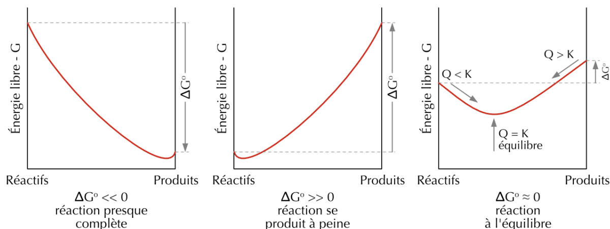
FIGURE 23.3 – Énergie libre standard et transformation spontanée
