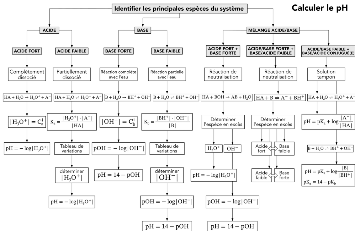
FIGURE 19.3 – Guide méthodologique pour la détermination du pH
