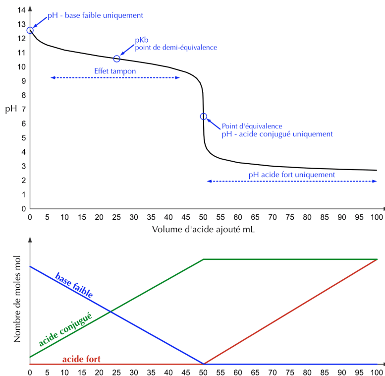
FIGURE 19.8 – Neutralisation d'une base faible par un acide fort
