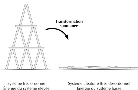
FIGURE 23.1 – Deuxième loi de la thermodynamique
