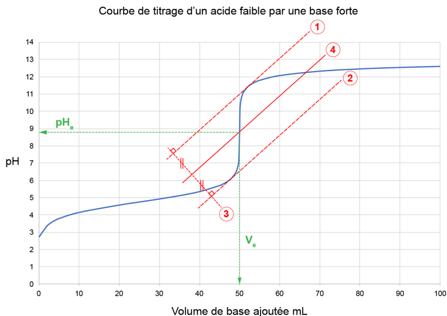
FIGURE 19.10 – Détermination graphique du point d'équivalence
