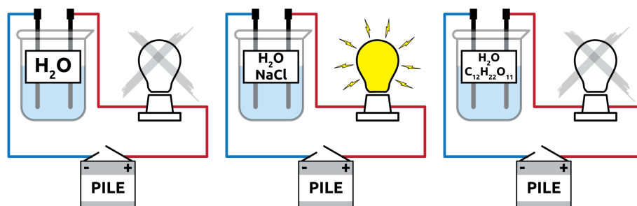
Figure 10.4: Conduction électrique des solutions (eau pure, solution de \text{NaCl} , solution de saccharose)
