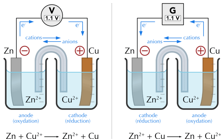
FIGURE 21.3 – Pile électrique et cellule électrolytique.
