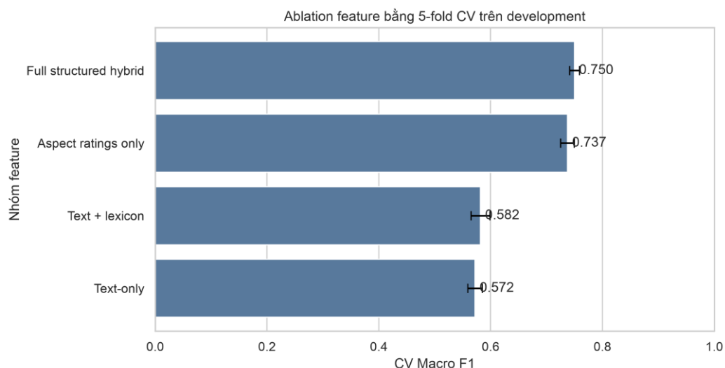
Hình 3.2. Macro F1 của các nhóm đặc trưng trong nghiên cứu loại bỏ
