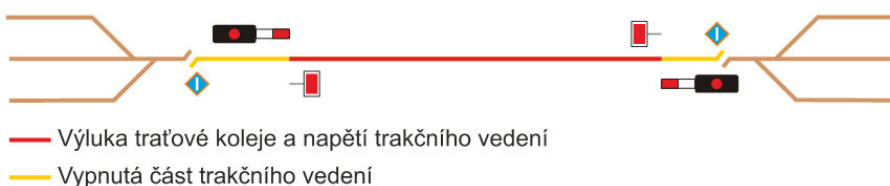
(9) Pokud je v dopravně s kolejovým rozvětvením prováděn pravidelný posunu, kdy posunový díl jede až za elektrické dělení, musí se přenosné návěstidlo s návěstí Stůj umístit na odjezdovém záhlaví v úrovni vjezdového návěstidla a před elektrickým dělením musí být umístěno přenosné návěstidlo nebo indikátor s návěstí Stáhněte sběrač (viz obrázek 246) na základě požadavku příslušné OSŘP, který musí být zpracován do VR.
