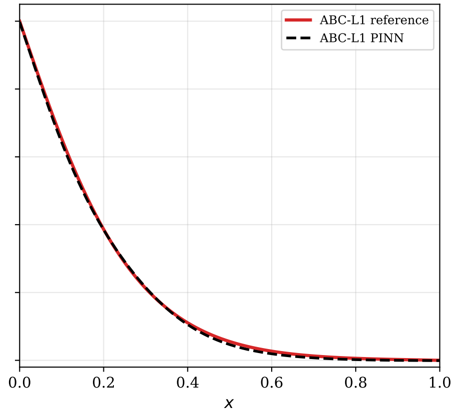
ABC-L1
