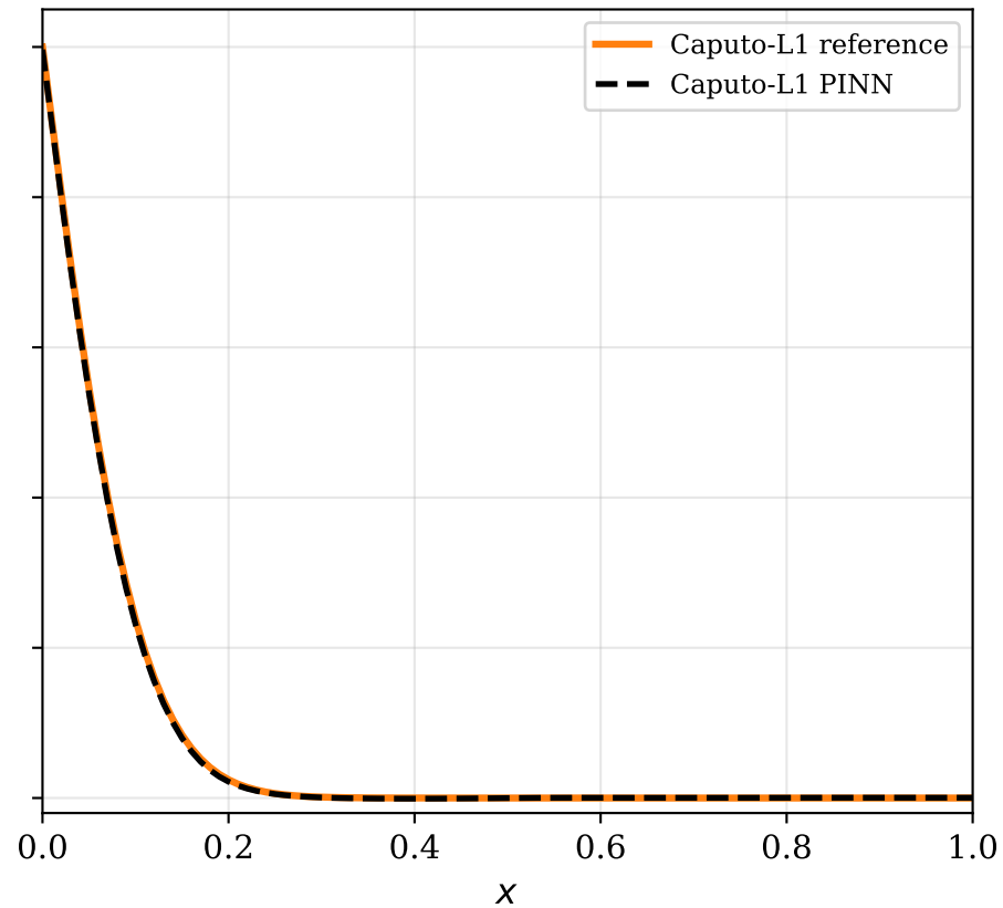
Caputo-L1
