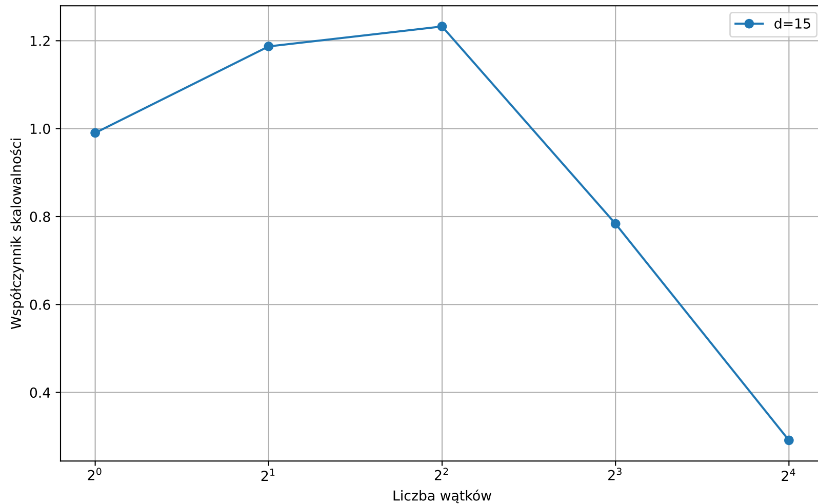
Skalowalność dla d=15
