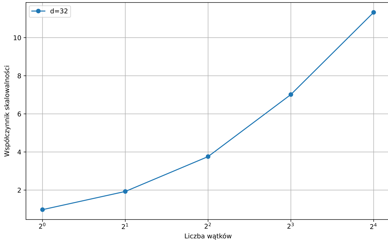
Skalowalność dla d=32
