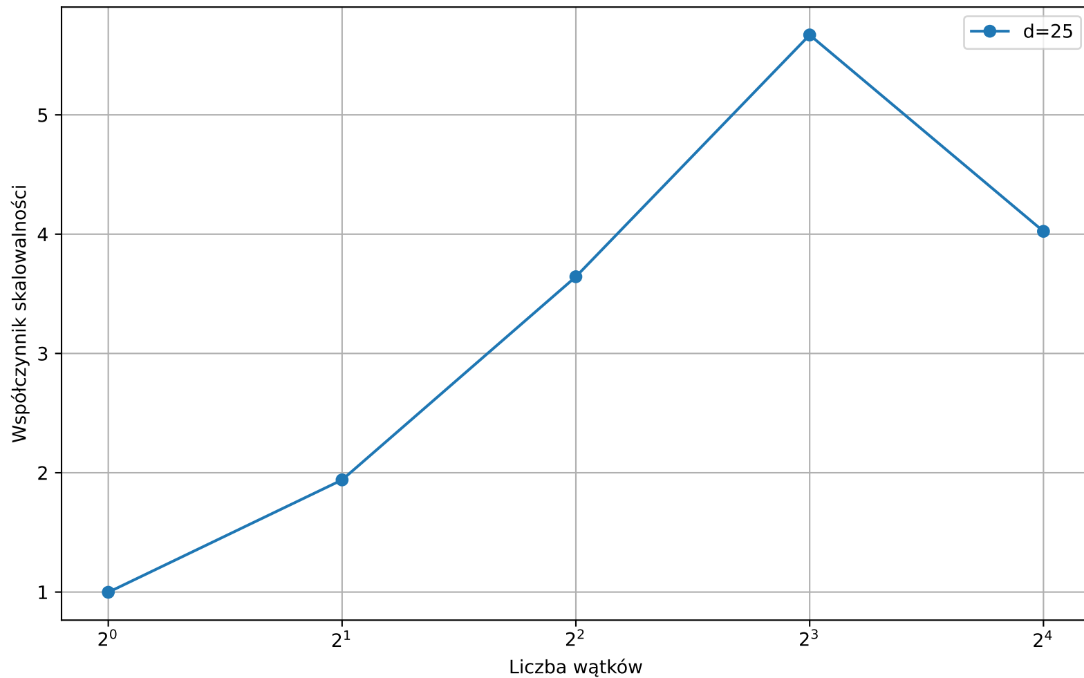
Skalowalność dla d=25
