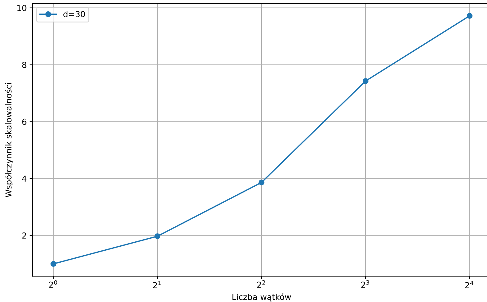
Skalowalność dla d=30
