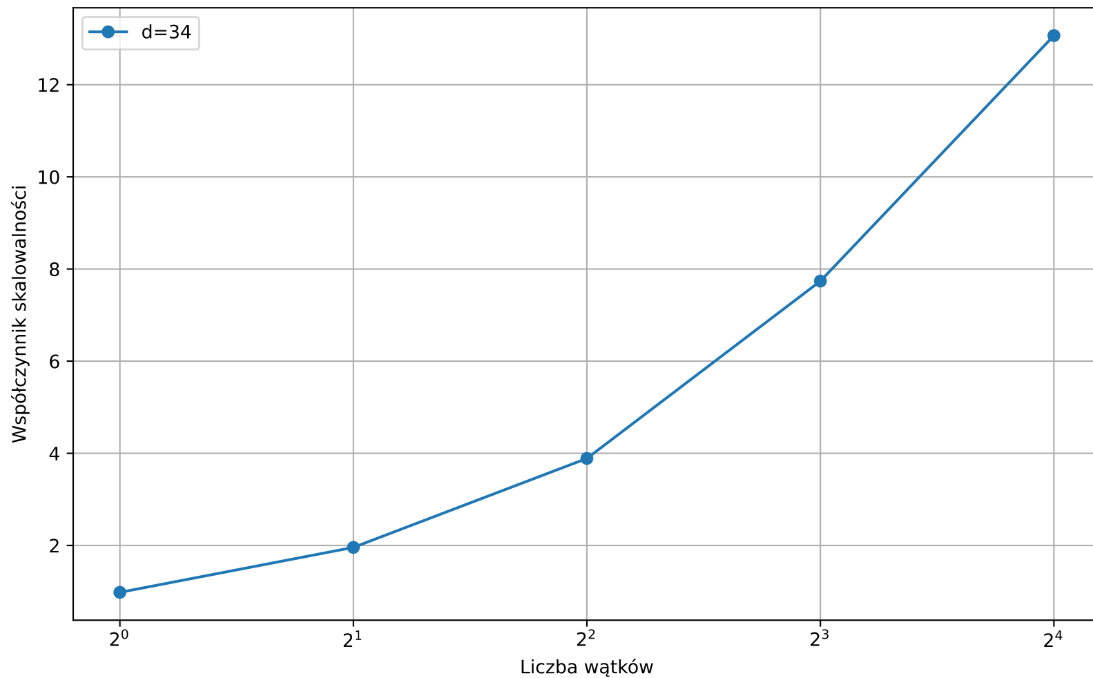
Skalowalność dla d=34
