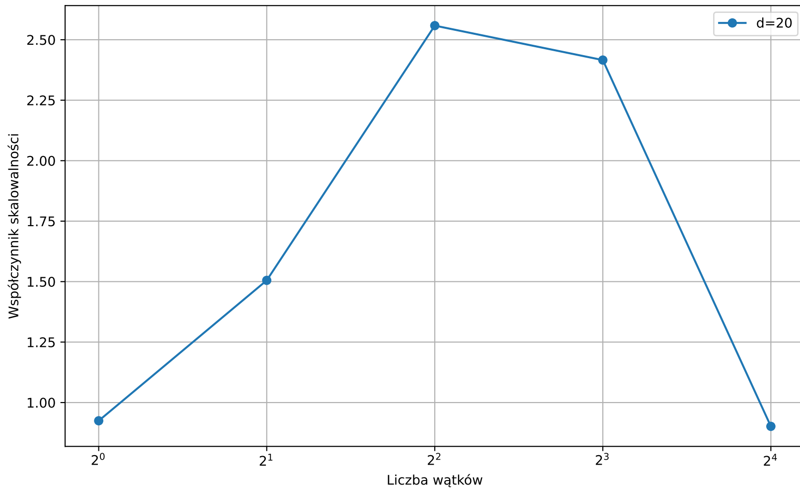
Skalowalność dla d=20
