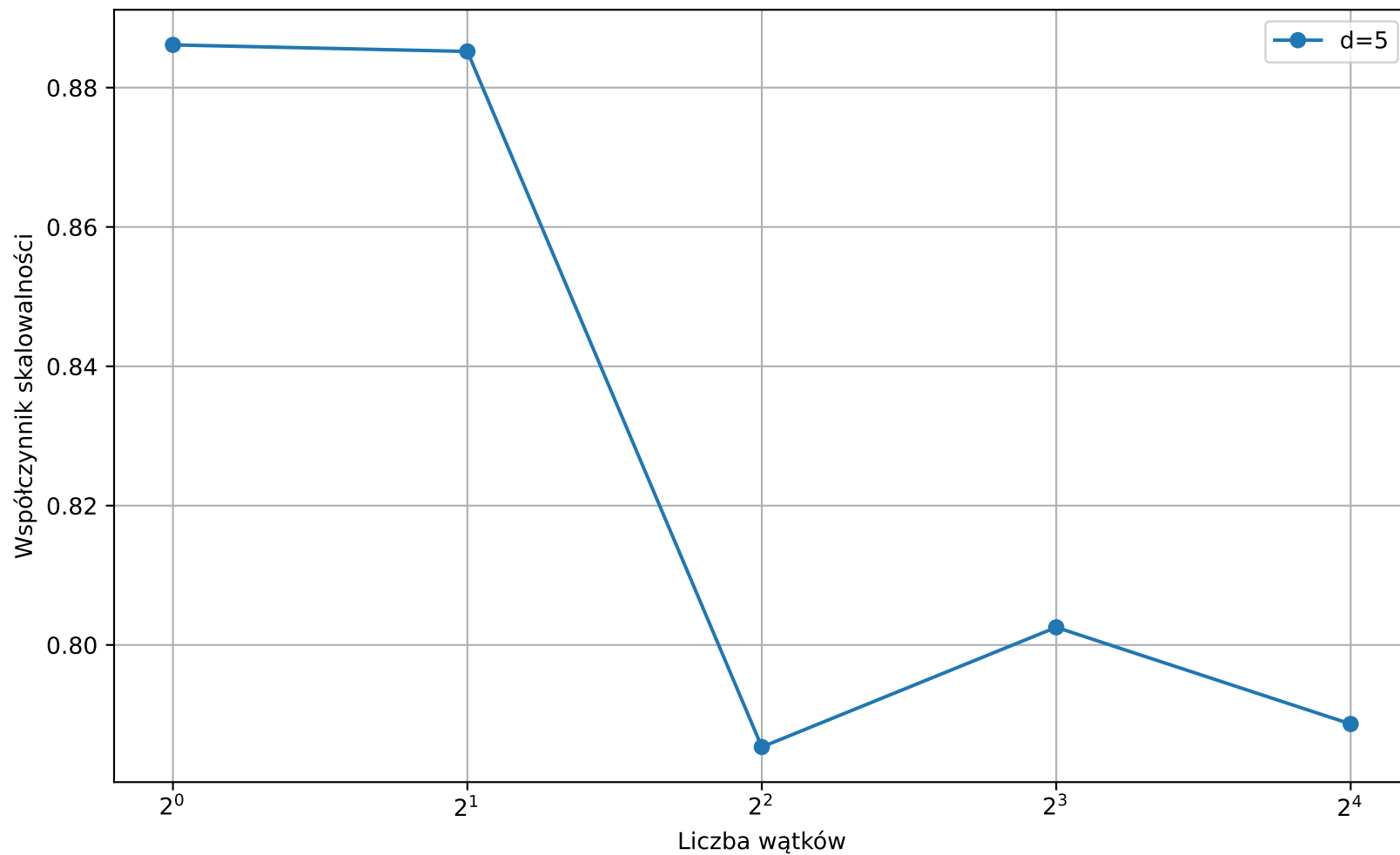
Skalowalność dla d=5
