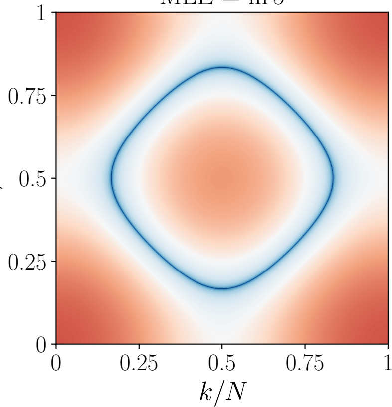
von Neumann MLE = \ln 5
