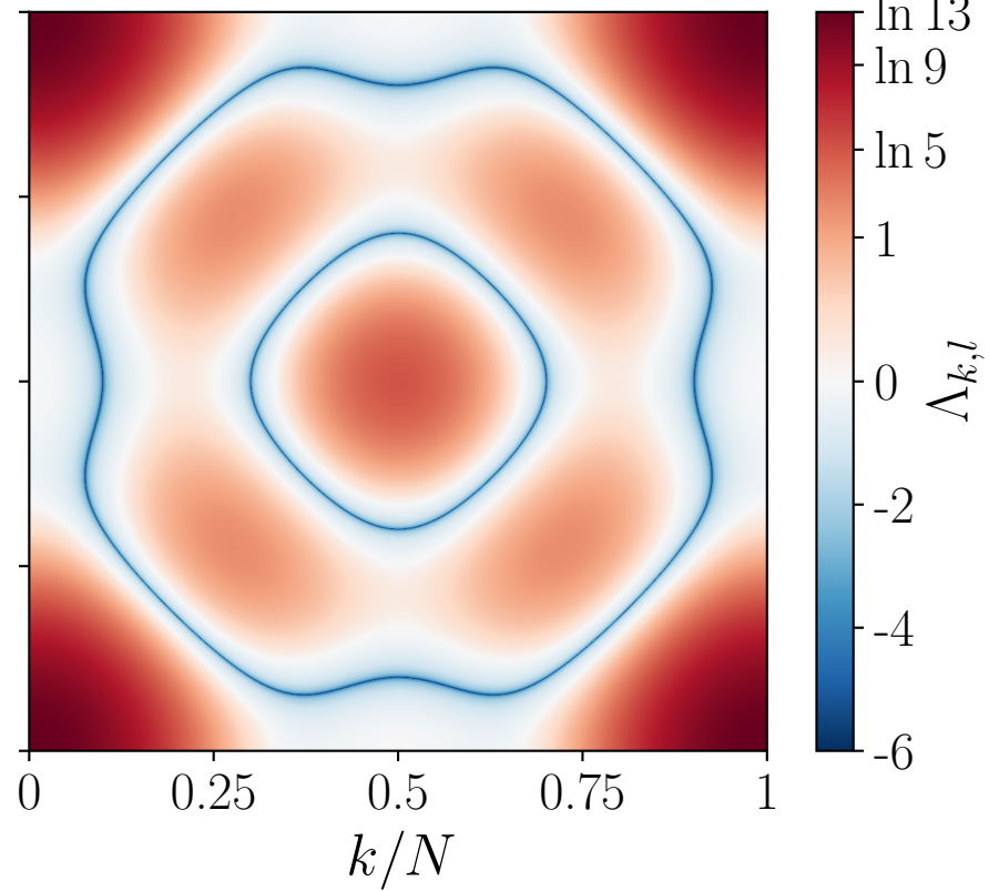
radius-2 von Neumann MLE = \ln 13
