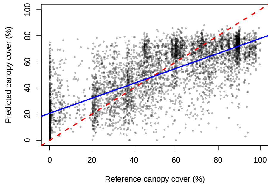
MLP
