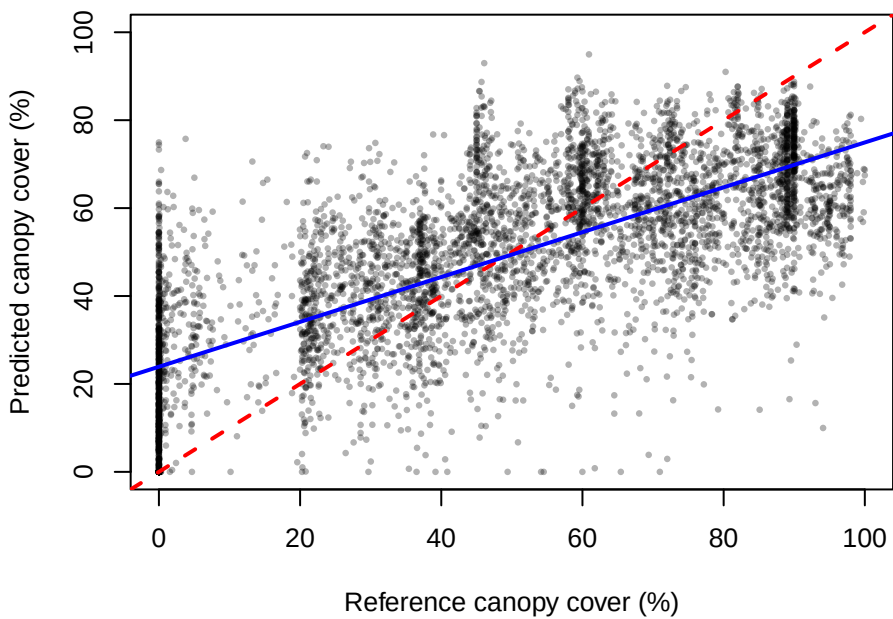
Linear regression
