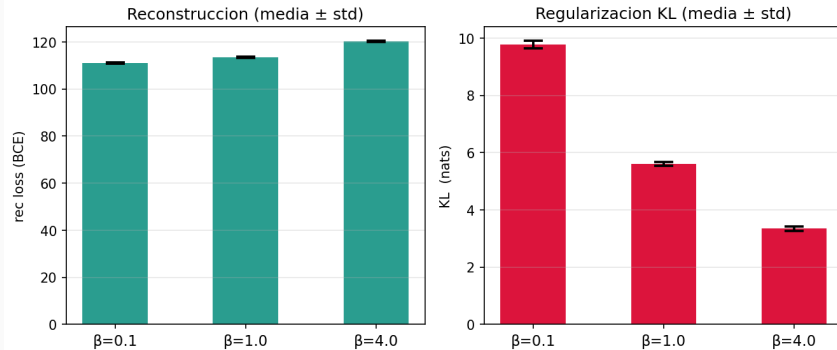
Estudio 2 — tradeoff rec/KL por \beta (5 seeds)
