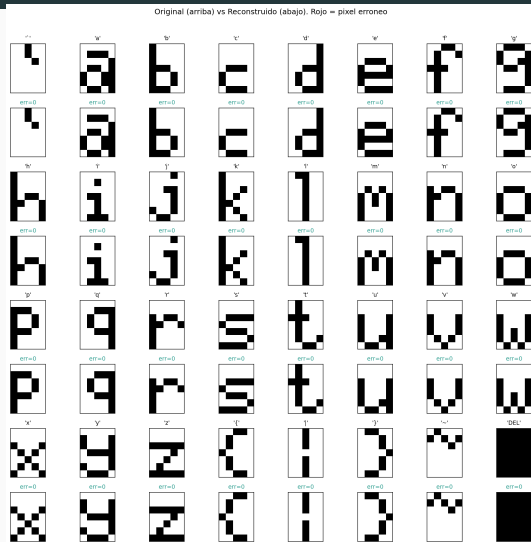
Original vs reconstruccion (32 letras).
