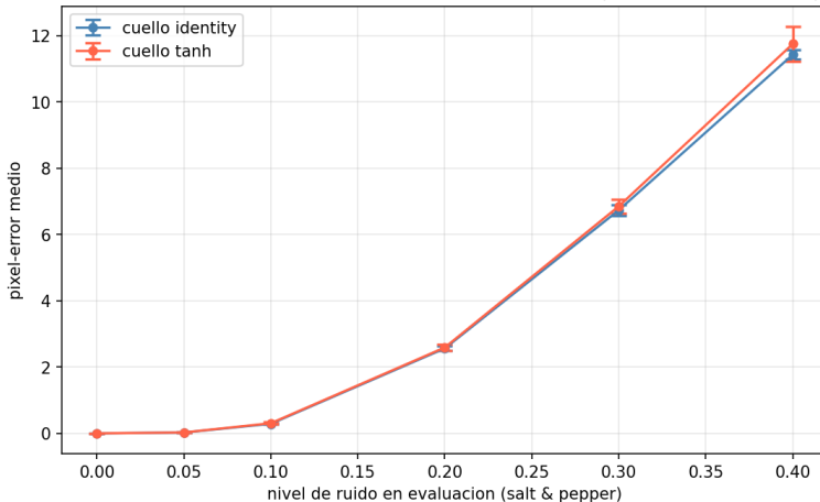
DAE cuello 8D: activacion del cuello identidad vs tanh (media \pm std, 5 seeds)
