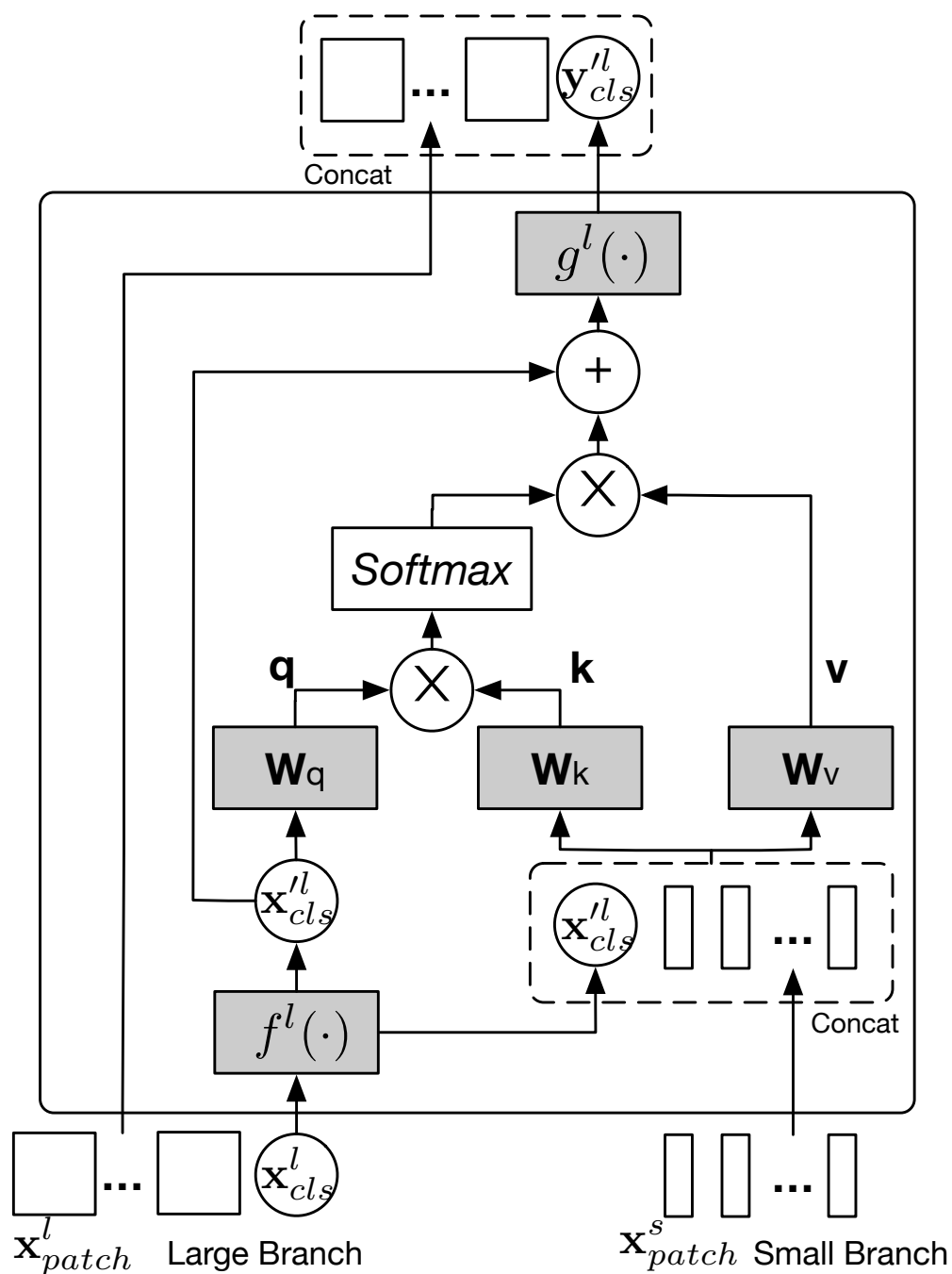
شکل ۱۱.۲: ماژول توجه متقابل در CrossViT: توکن کلاس یک شاخه نقش پرس و جو را دارد و اطلاعات را از توکن های شاخه دیگر دریافت می کند [۵].
