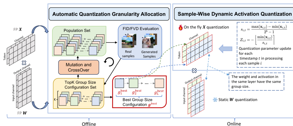
شکل ۶.۲: شماتیک روش کوانتیزاسیون در Q-DiT [۷۲].
