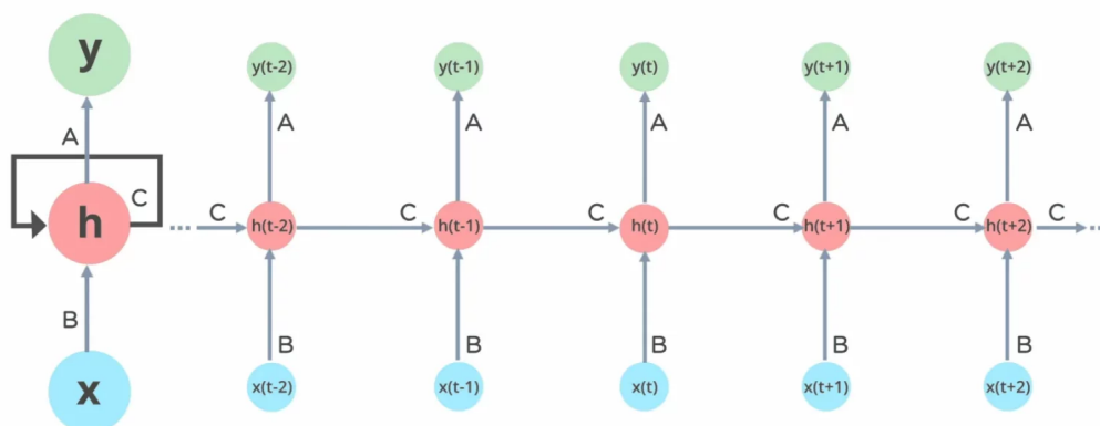
شکل ۲.۱: معماری شبکه عصبی بازگشتی (RNN) و نحوه باز شدن آن در طول زمان.
