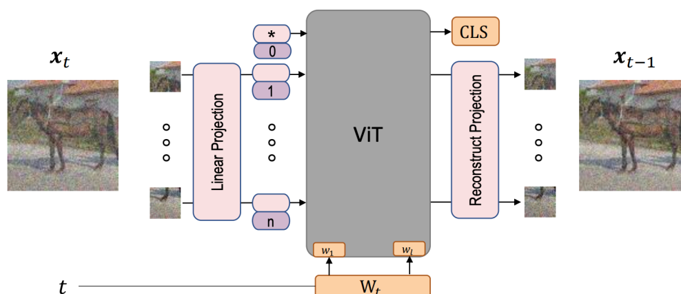
شکل ۱.۲: معماری GenViT که مبدل را در مدل انتشار ادغام می‌کند.
