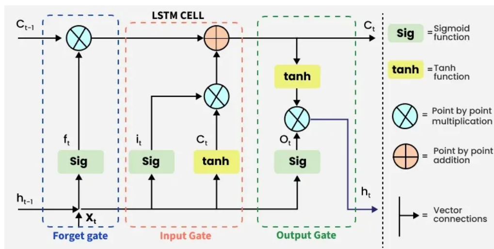
شکل ۳.۱: ساختار داخلی یک واحد LSTM شامل دروازه‌های فراموشی، ورودی و خروجی.
