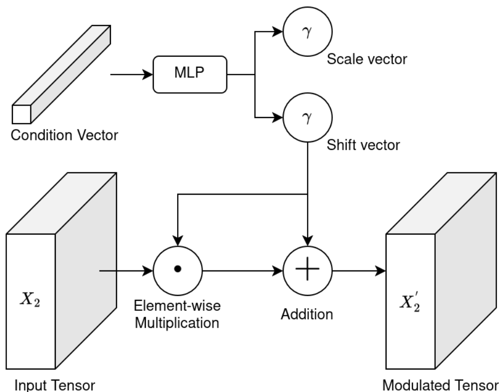
شکل ۵.۳: بلوک شرط‌گذاری FiLM. بردار شرط c پارامترهای مقیاس و انتقال را تولید می‌کند که بر روی ورودی اعمال می‌شوند.
