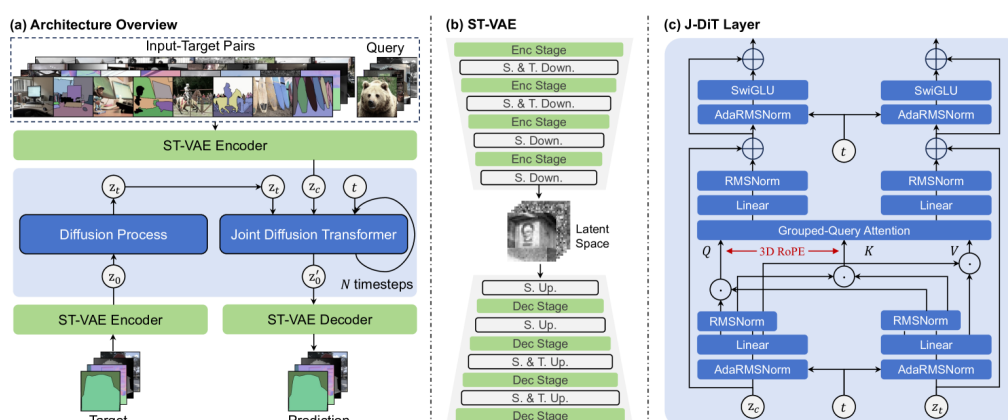
شکل ۵.۲: معماری پیشنهادی در LaVin-DiT برای بهبود مقیاس‌پذیری [۷۱].
