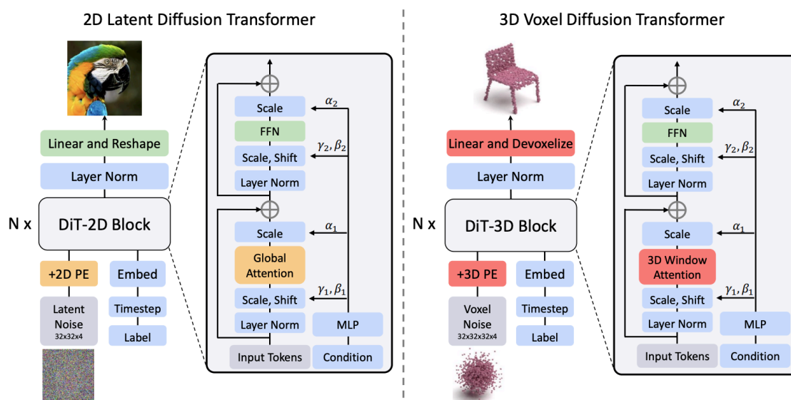
شکل ۷.۲: معماری DiT-3D: تعمیم مکانیزم پیچ‌سازی و توجه به فضای حجمی برای تولید سه‌بعدی [۴۲].
