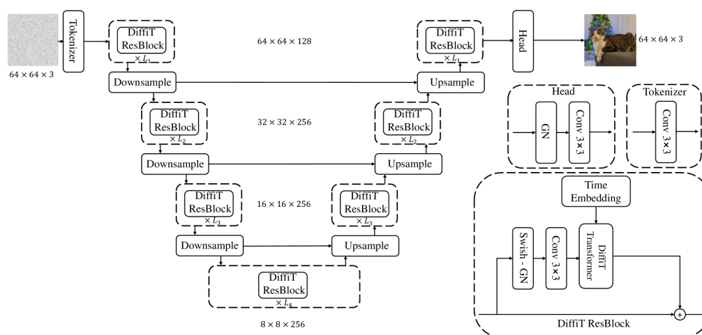
شکل ۴.۲: معماری DiffiT با بلوک‌های توجه وابسته به زمان (TMSA).
