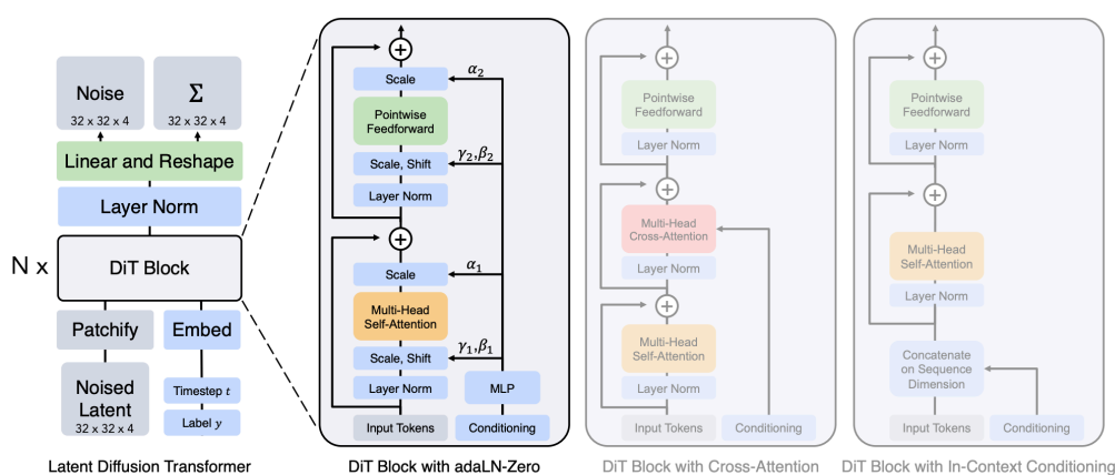
شکل ۳.۲: معماری DiT مبتنی بر بلوک‌های استاندارد مبدل و adaLN.
