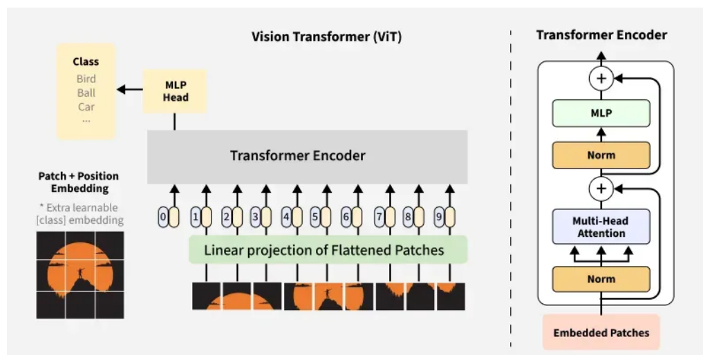
شکل ۵.۱: معماری مبدل بینایی (ViT) شامل تقسیم تصویر به تکه‌ها، تعبیه خطی و رمزگذار مبدل.
