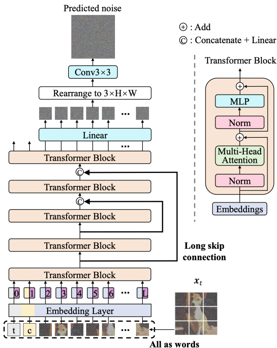
شکل ۲.۲: معماری U-ViT با اتصالات پرشی بلند بین بلوک‌های مبدل [۱].
