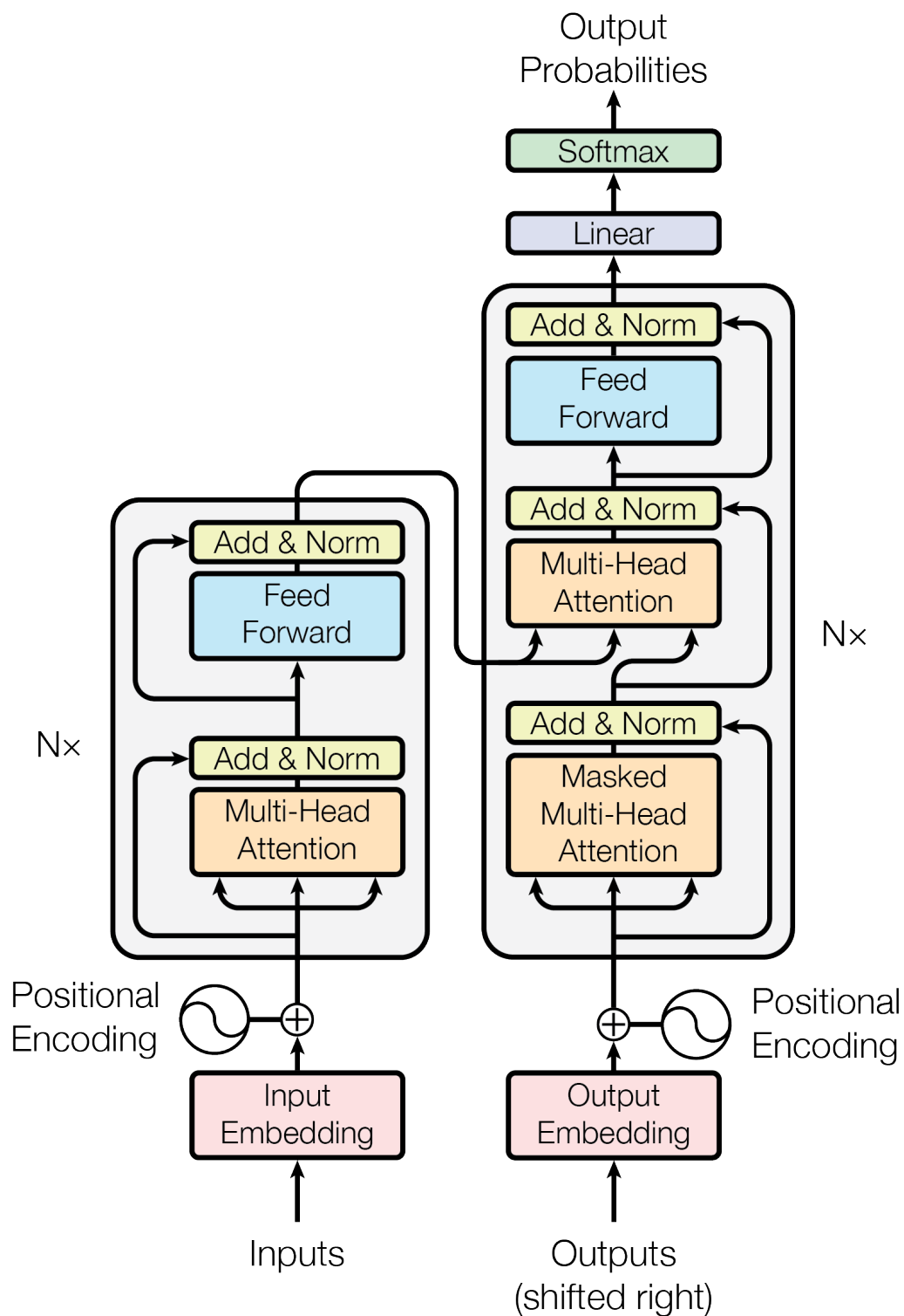
شکل ۴.۱: ساختار کلی معماری مبدل شامل رمزگذار و رمزگشا.
