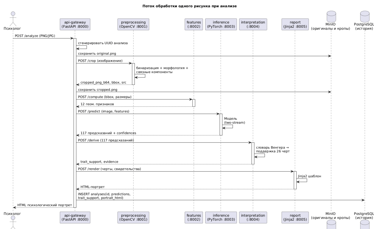
Рисунок 6 - Поток обработки одного рисунка при анализе: последовательность вызовов между микросервисами, MinIO и PostgreSQL
