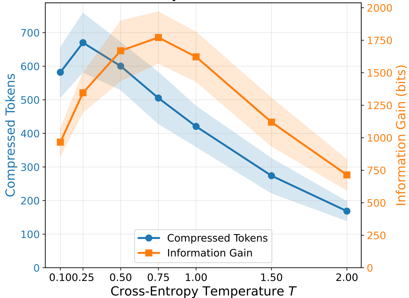
Pythia-1.4b
