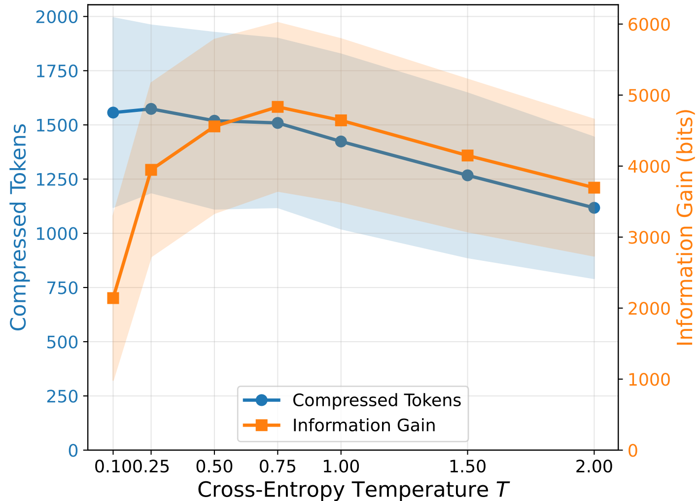
Llama-3.1-8B
