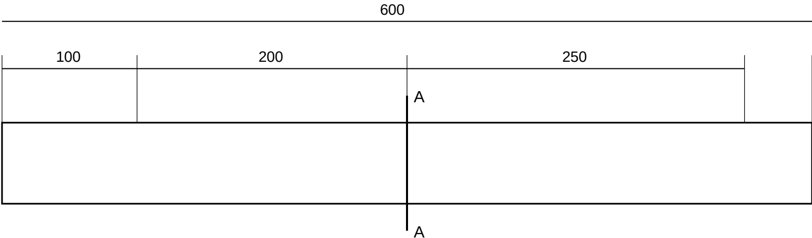
PLANTA VIGA V-12 ESC 1:50
