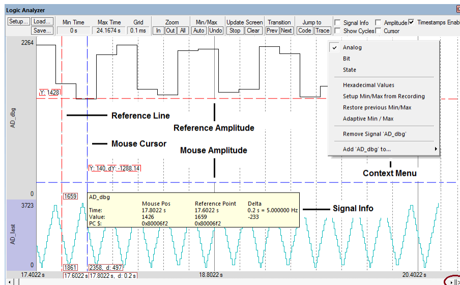
Fig. 4.1: Analizador lógico de ARM Keil Microvision.
