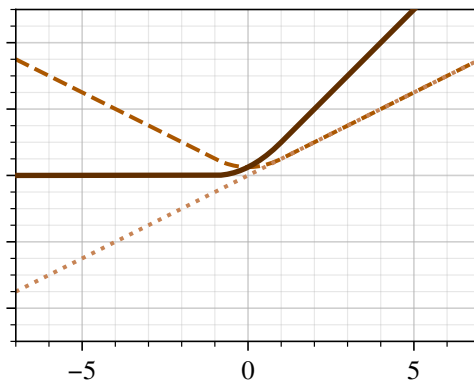
sparse_plus
