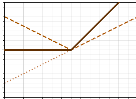
sparse_plus
