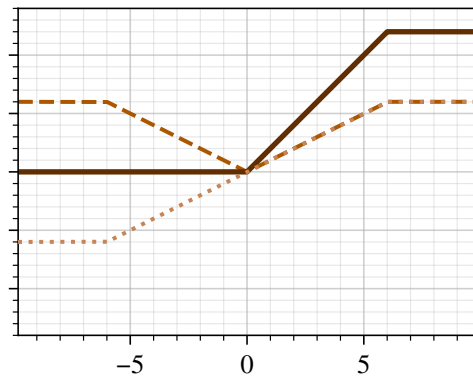
relu6
