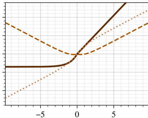
selu
