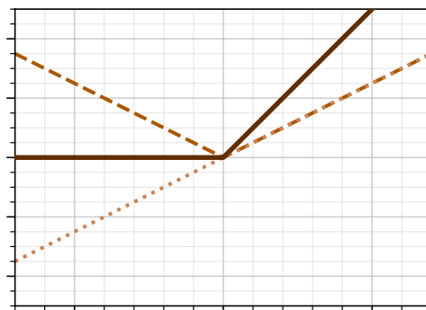
sparse_plus
