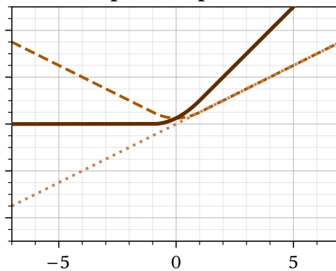
sparse_plus
