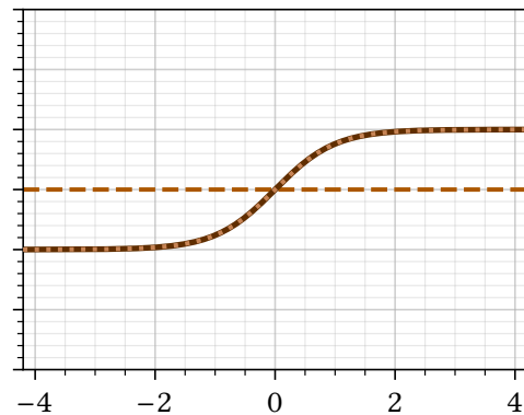
tanh
