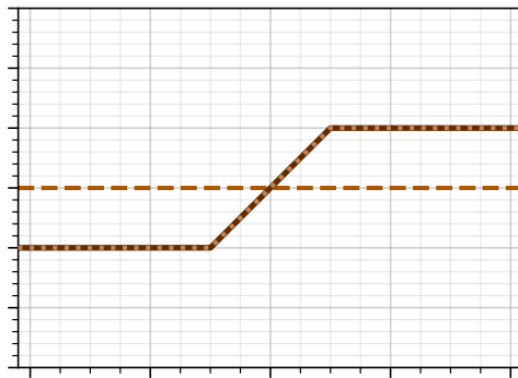
sparse_sigmoid
