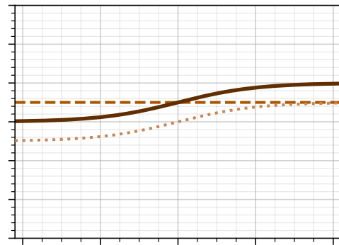
tanh
