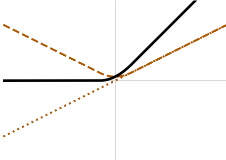
Sparseplus
